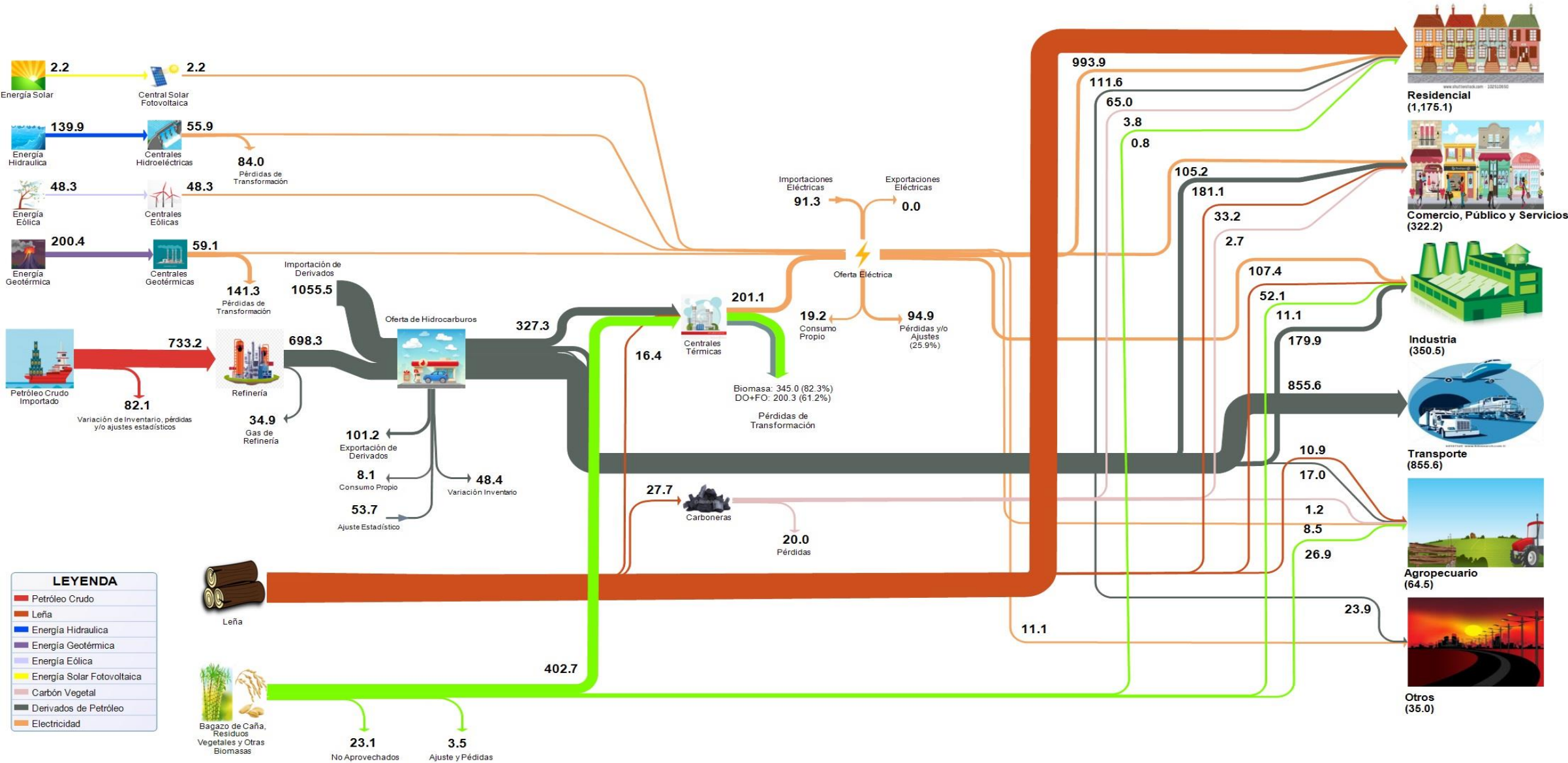
Figura no. 1 Flujo de Energía (cifras en miles de tep)
