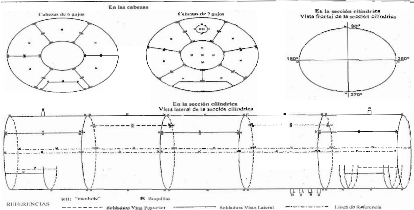
Figura No. 6 Tipo de Rotulación para Cisternas
